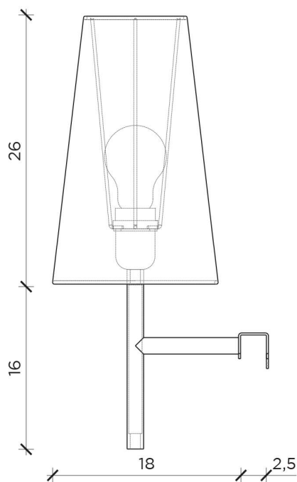
LATO | SIDE
