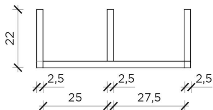
PIANTA | PLAN
