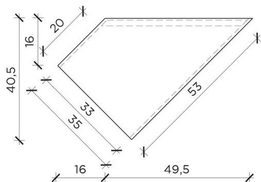
PIANTA | PLAN
