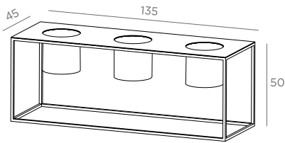
VASO RIVIERA 3 FIORI 50 POT RIVIERA 3 FIORI 50
