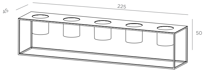
VASO RIVIERA 5 FIORI 50 POT RIVIERA 5 FIORI 50
