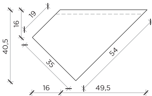
PIANTA | PLAN
