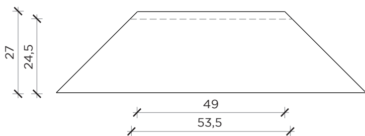
PIANTA | PLAN
