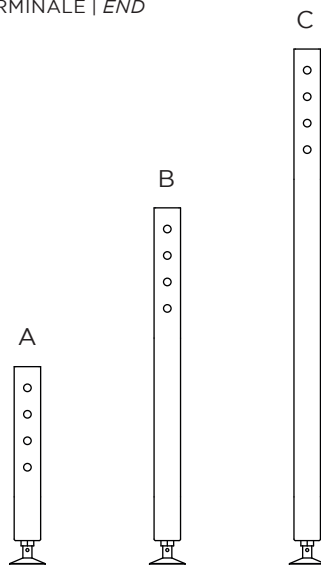
TERMINALE | END
